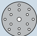
GLS 47 ø 150 mm 8 otworów odpylających ø 9 mm na obwodzie ø 120 mm, 6 otworów odpylających ø 9 mm na obwodzie ø 80 mm + 1 otwór środkowy ø 17 mm
